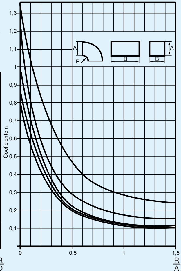
Sección rectangular
