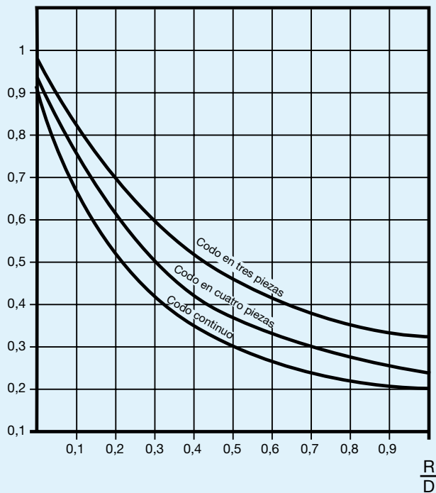
Sección circular
