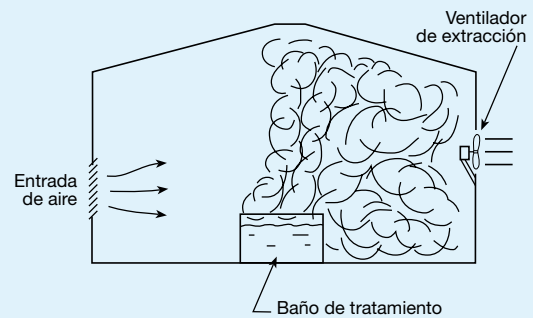
Fig. 2.7: Los dos grandes tipos de ventilación.
