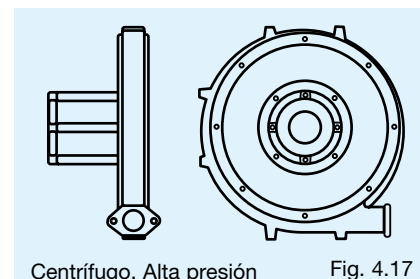
Centrífugo. Alta presión Fig. 4.17
